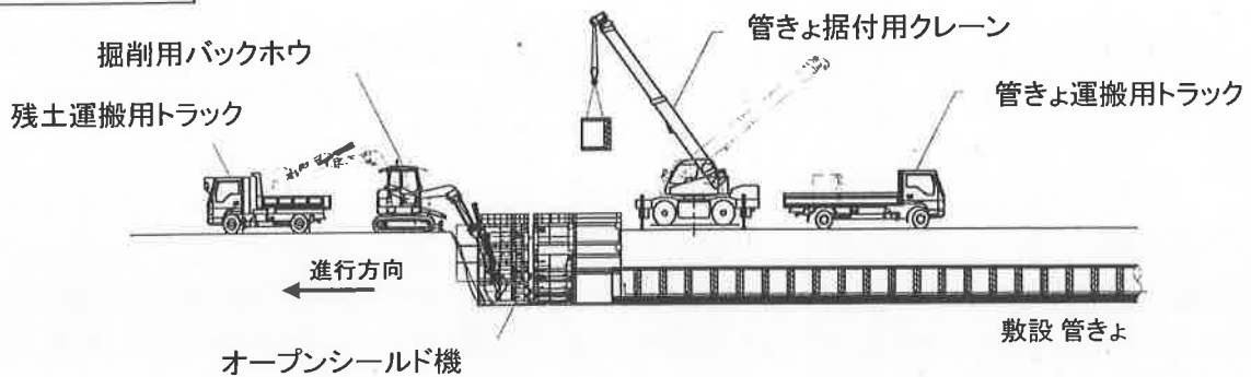
施工状況図
