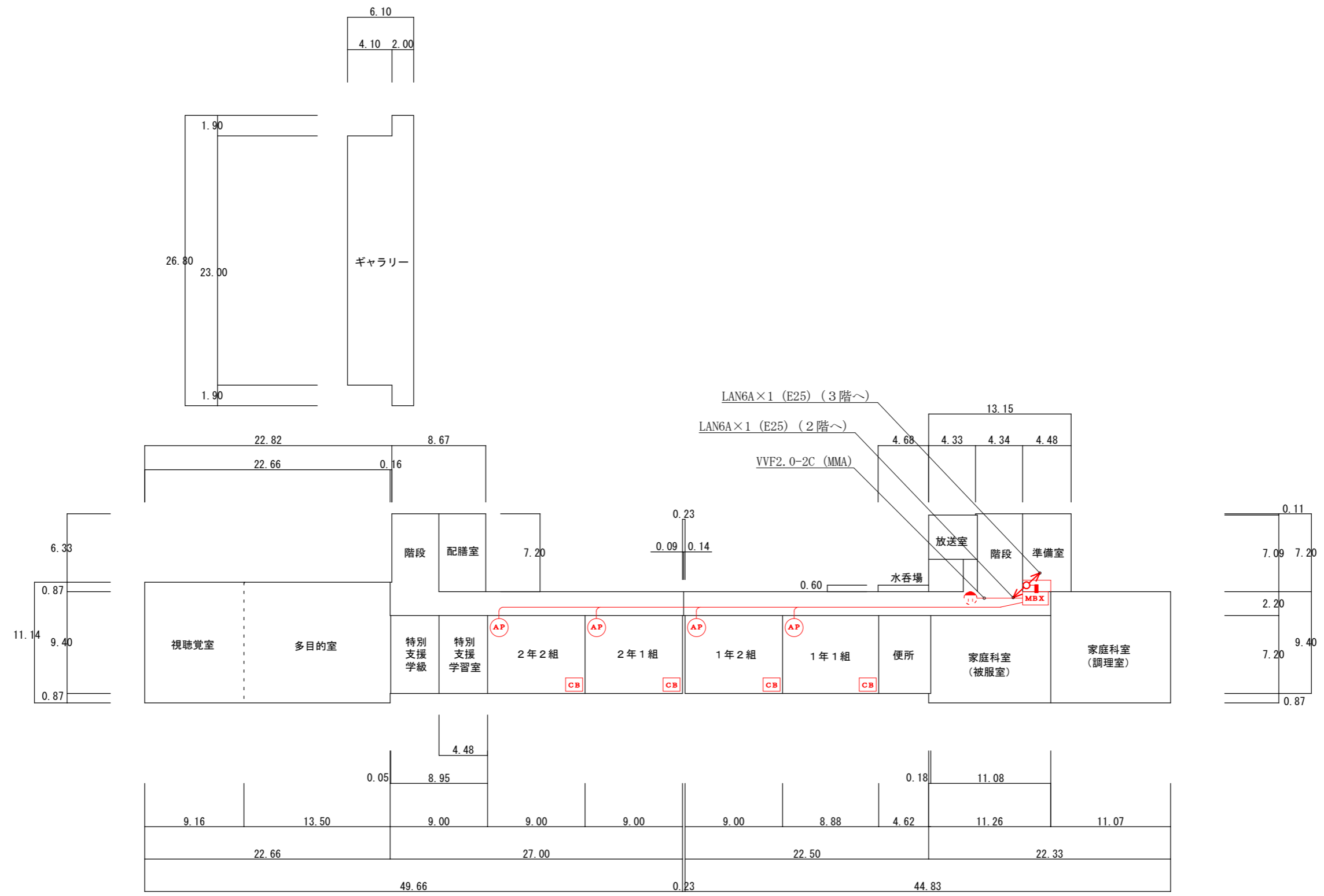
2階平面図
