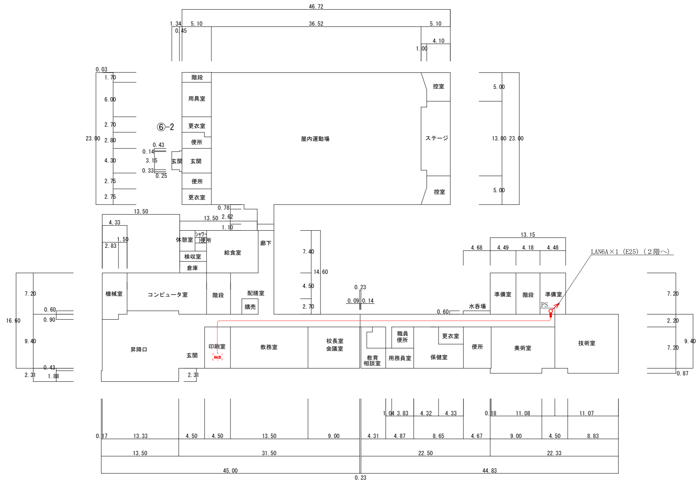
1階平面図
