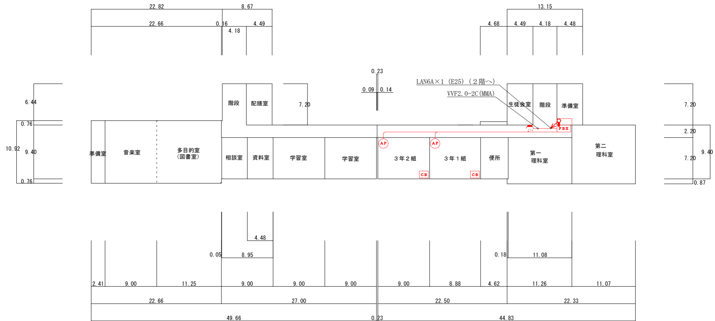
3階平面図
