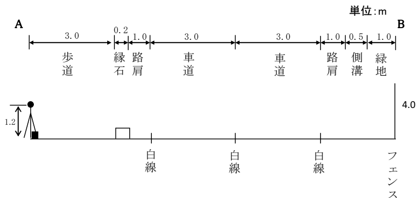
図 5-2-14(3) 道路構造（上千原地点）
