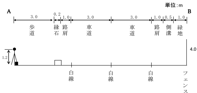
図 5-2-14(2) 道路構造（東中島地点）
