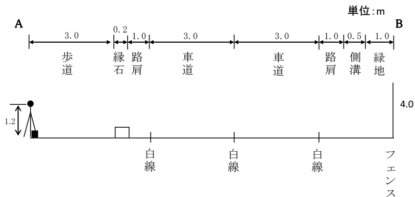
図 5-2-14(1) 道路構造（若鷹地点）
