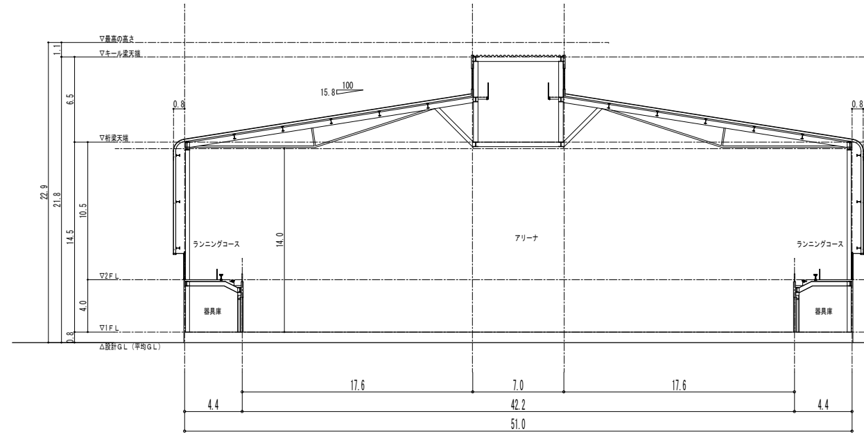
西-東 断面図
