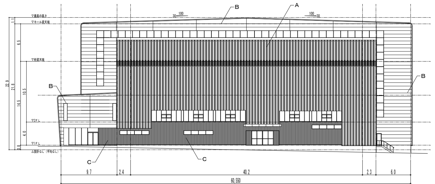
東側立面図
