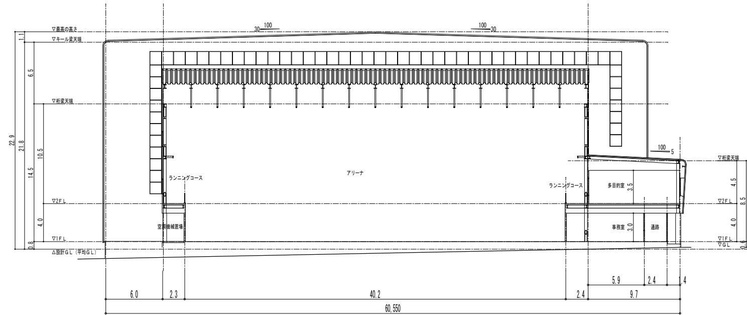
南-北 断面図
