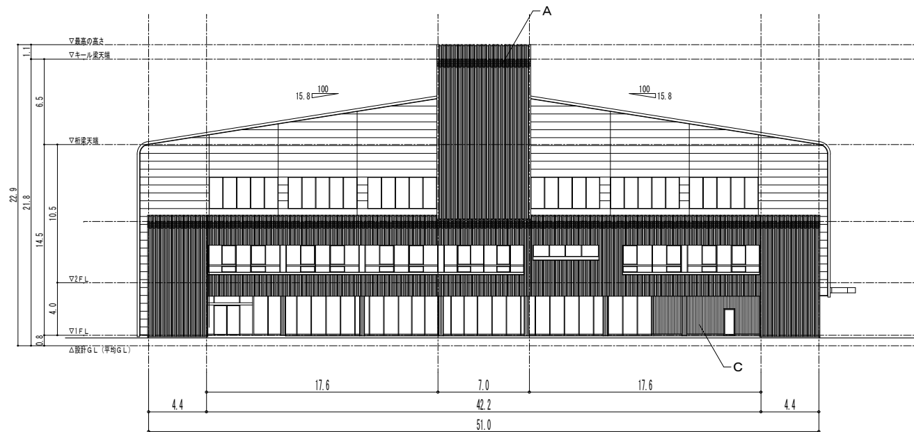
南側立面図
