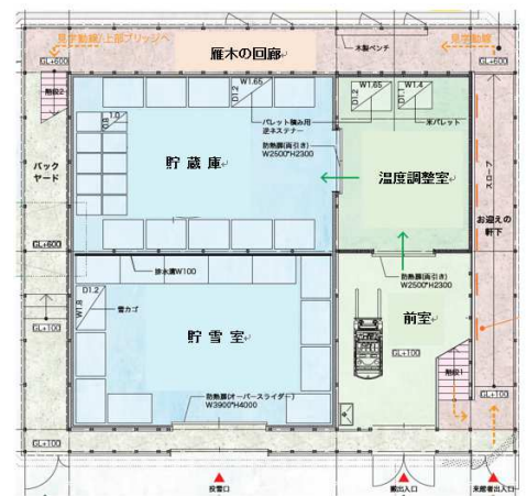
<1階 平面図>
