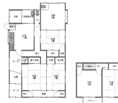
間取り
