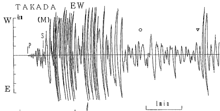
↓ (資料No.1-3) 東西方向の動きの波形
