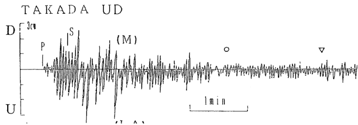
↑ (資料No.1-1) 上下動の波形
