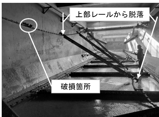
▲フライト板の脱落・破損
