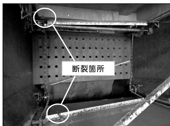
▲掻寄チェーンの断裂
