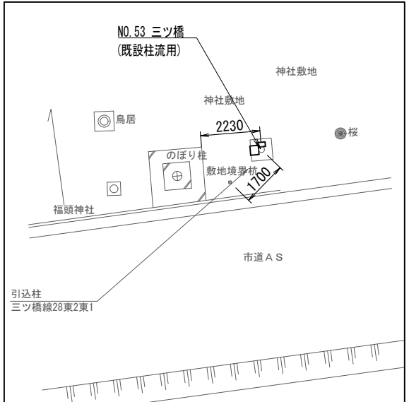
配置図 S=1/200
