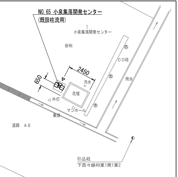
配置図 S=1/200
