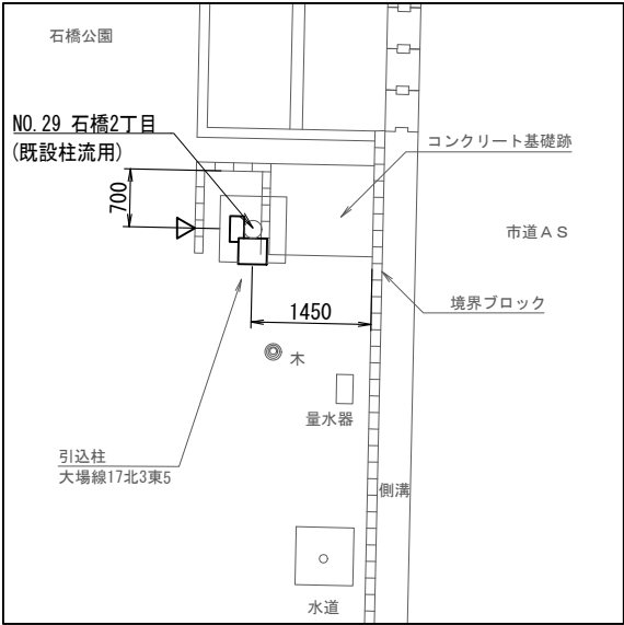
配置図 S=1/100
