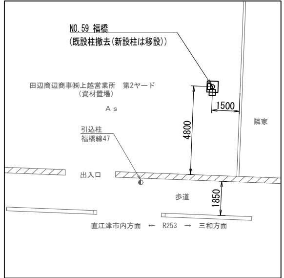
配置図 S=1/200
