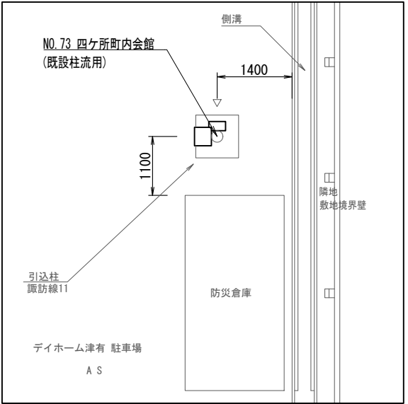
配置図 S=1/100
