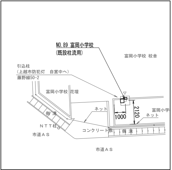
配置図 S=1/200
