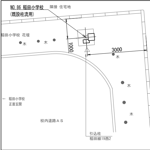
配置図 S=1/100
