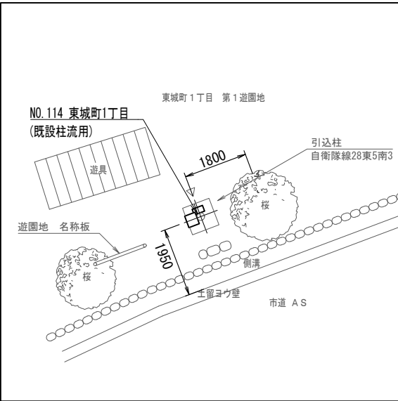
配置図 S=1/150
