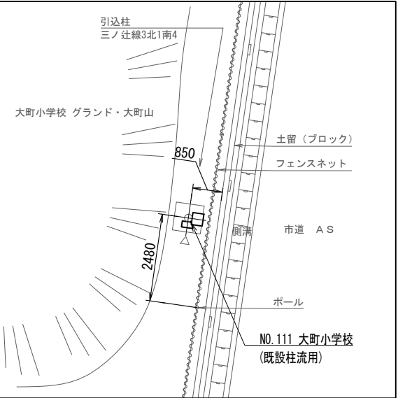
配置図 S=1/150
