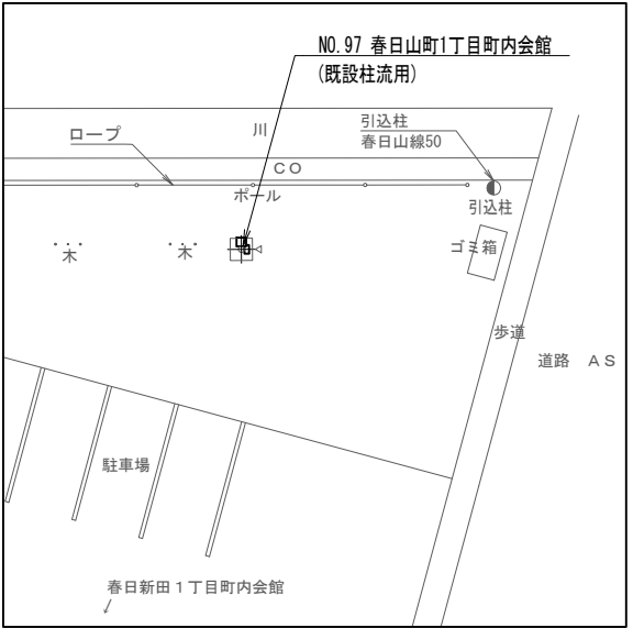
配置図 S=1/300
