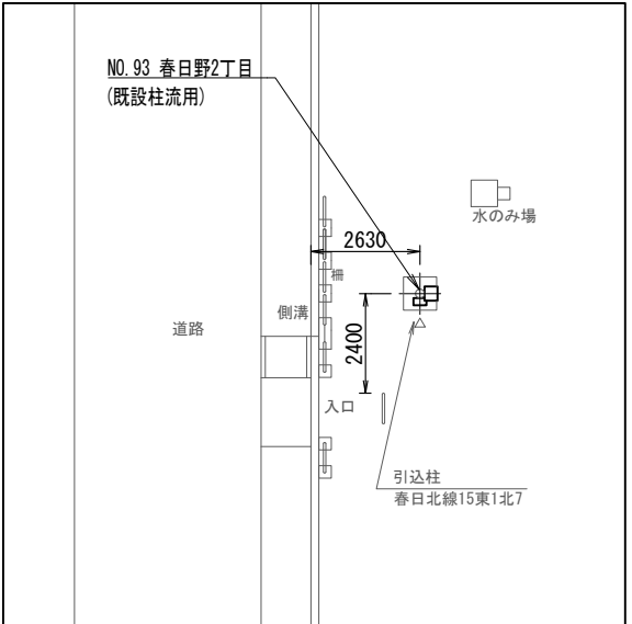
配置図 S=1/200
