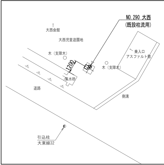
配置図 S=1/200
