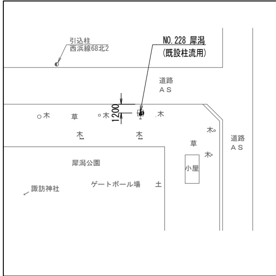
配置図 S=1/500
