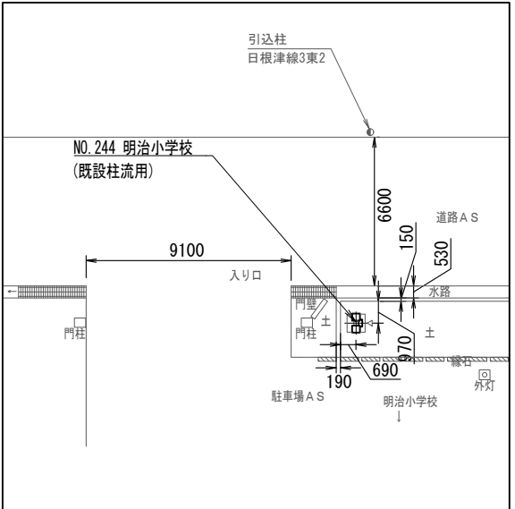
配置図 S=1/300
