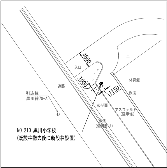
配置図 S=1/600
