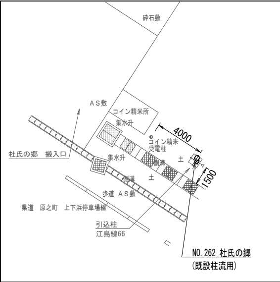
配置図 S=1/300
