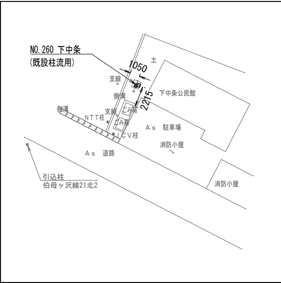
配置図 S=1/400
