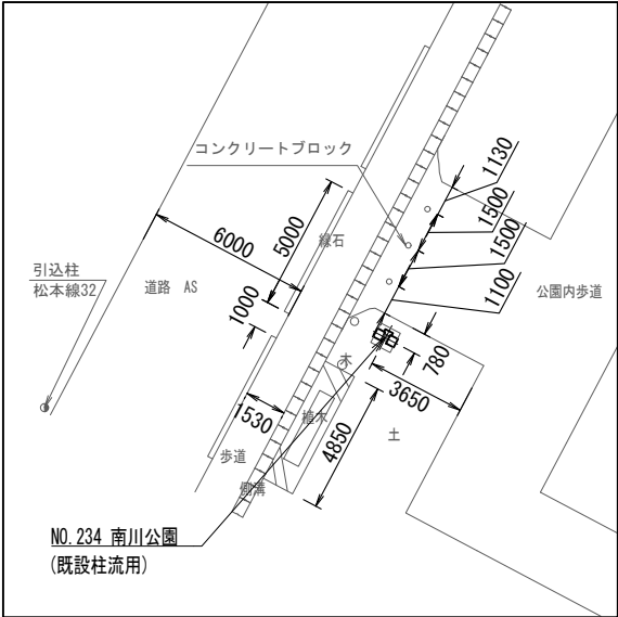
配置図 S=1/300
