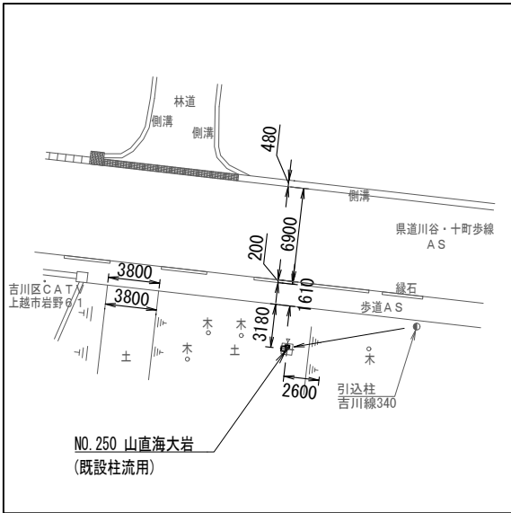
配置図 S=1/500
