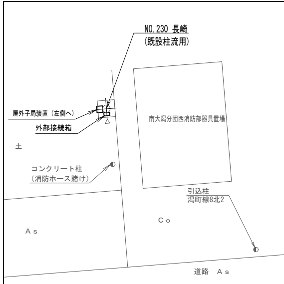
配置図 S=1/200
