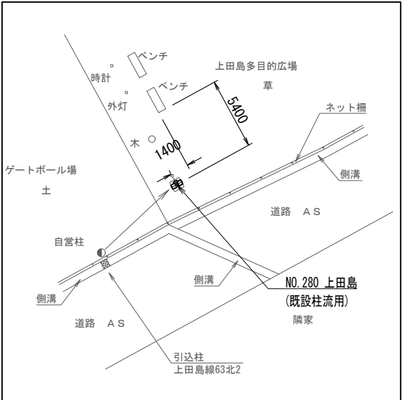
配置図 S=1/400
