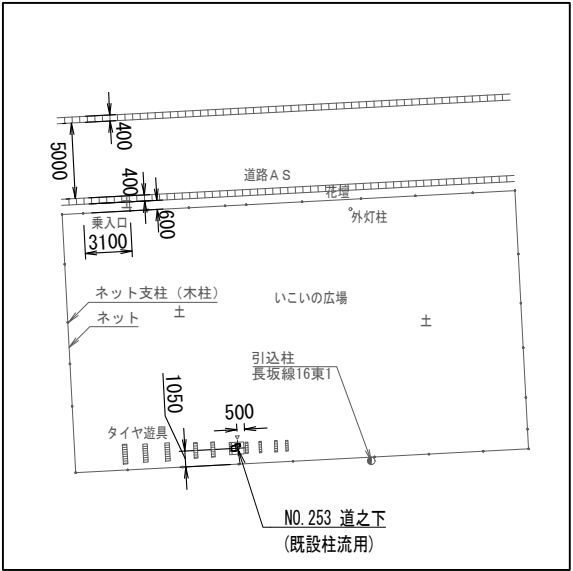
配置図 S=1/500
