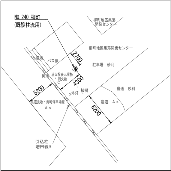
配置図 S=1/400
