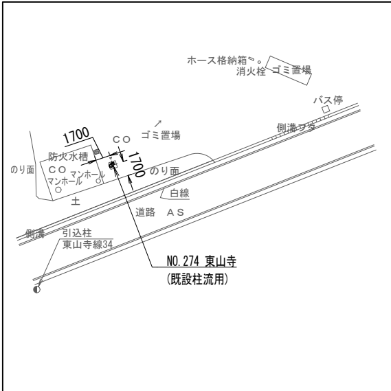
配置図 S=1/600
