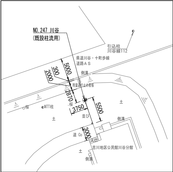
配置図 S=1/500
