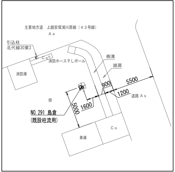
配置図 S=1/300
