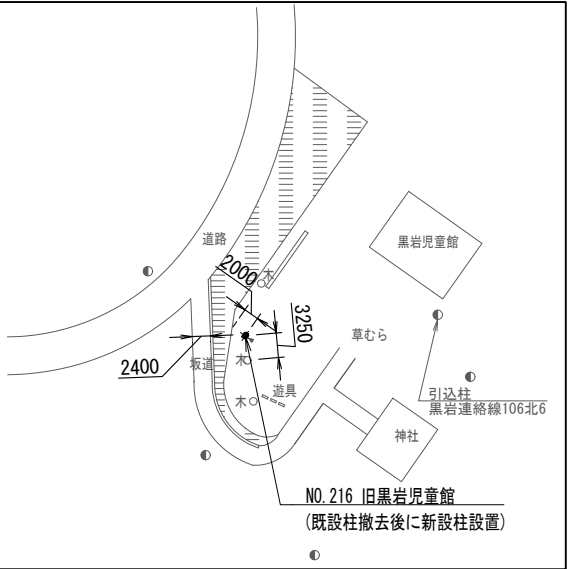
配置図 S=1/1000
