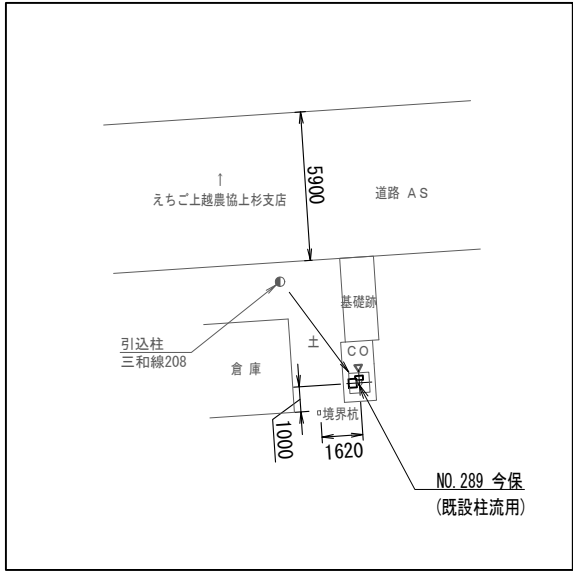
配置図 S=1/300
