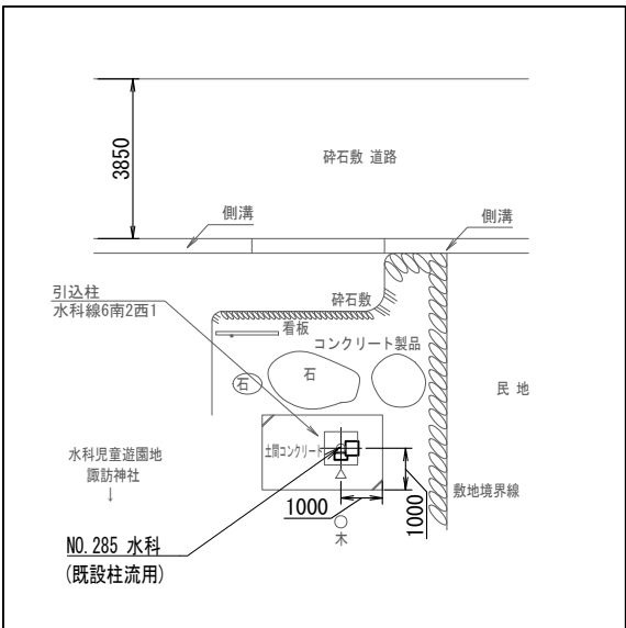
配置図 S=1/200
