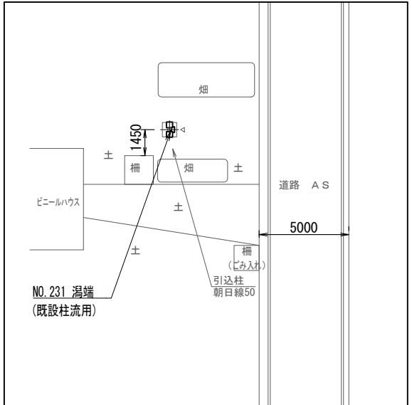
配置図 S=1/300
