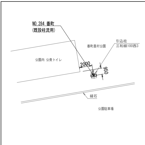
配置図 S=1/300
