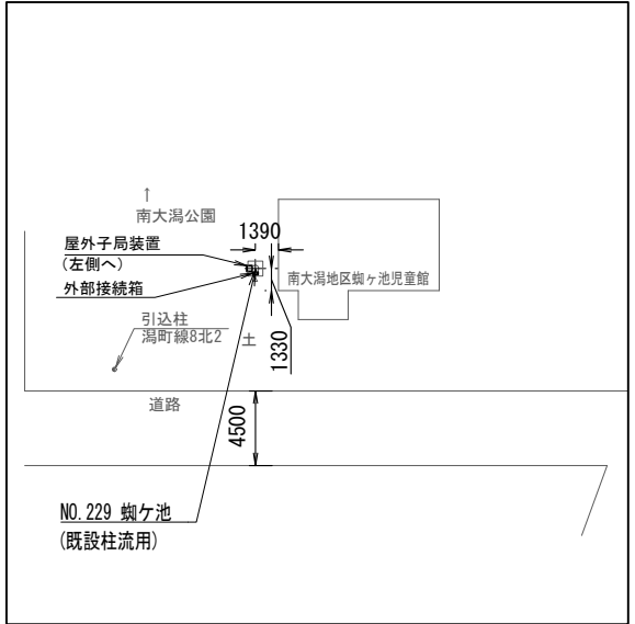
配置図 S=1/500
