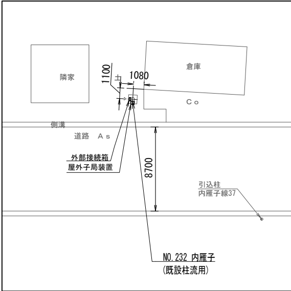
配置図 S=1/400
