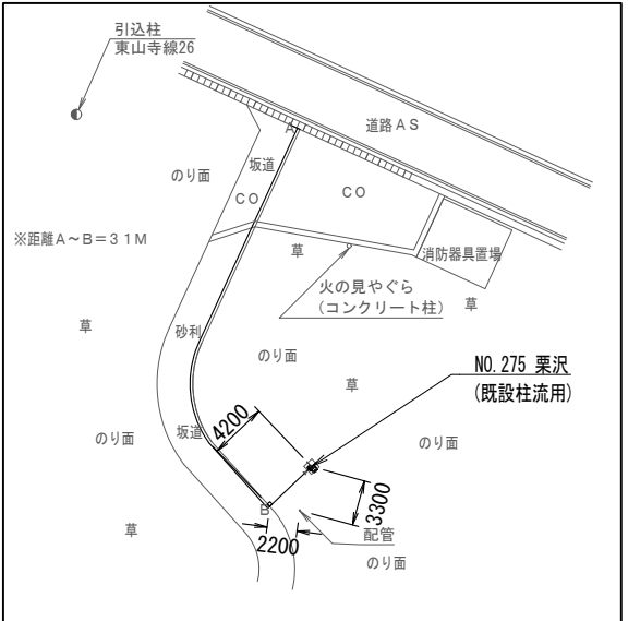
配置図 S=1/600
