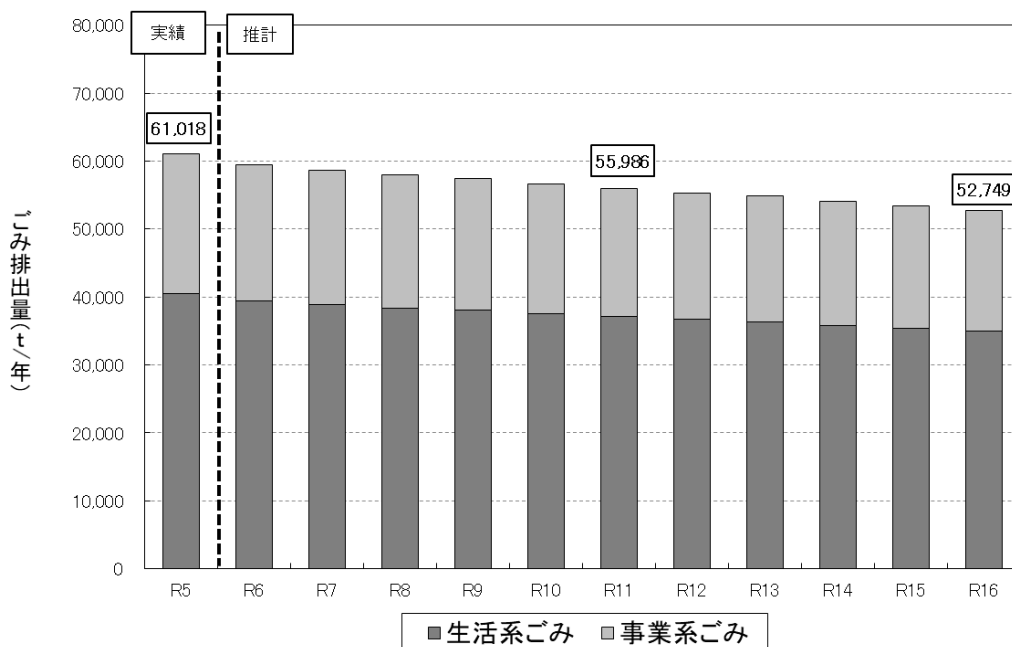
図 2-9 ごみ総排出量の将来予測結果
