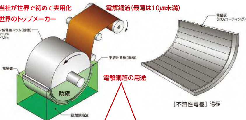
【電解銅箔製造用装置概略図】
