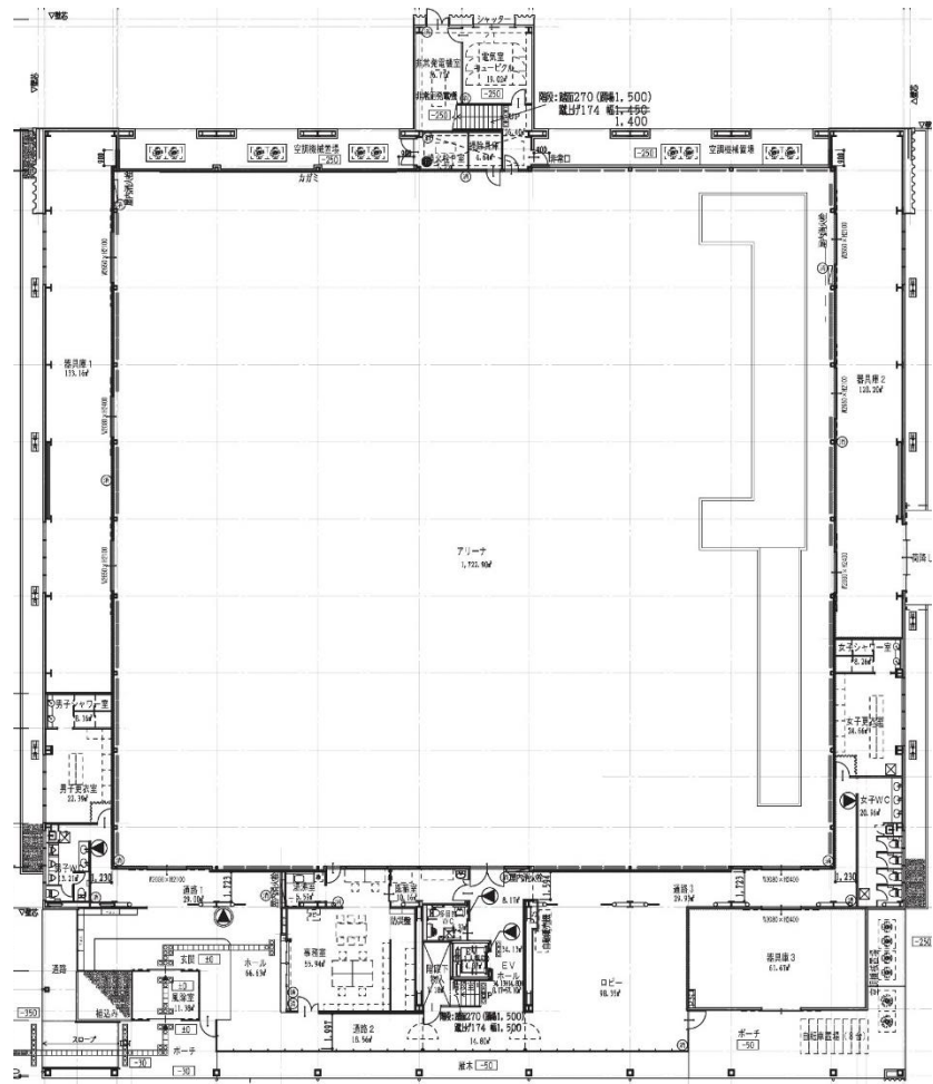
上越市立上越体操場 1階ロビー図
