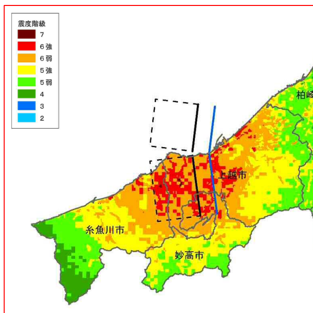
震度分布図 高田平野西縁断層
