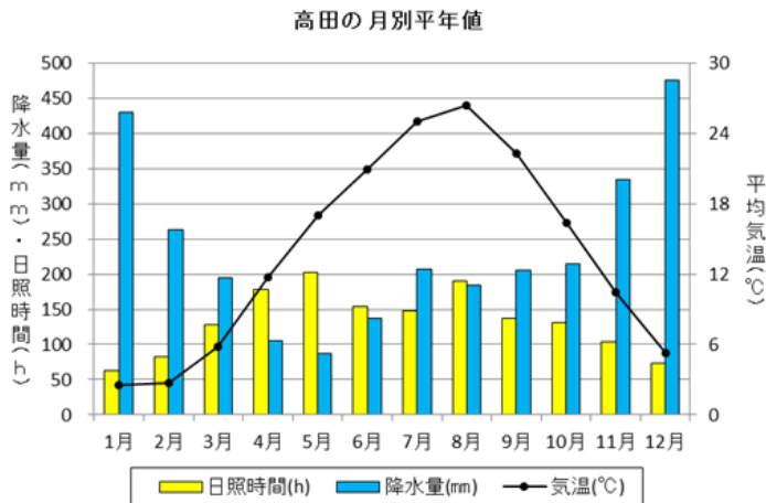
市内アメダス地点の月別平年値
