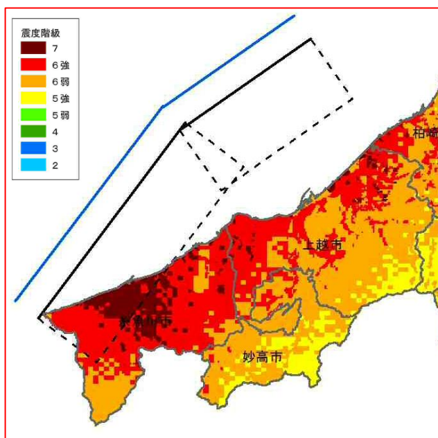
震度分布図 F41（上越・糸魚川沖）
