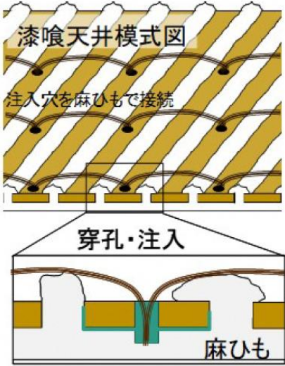
▲技術概要図
