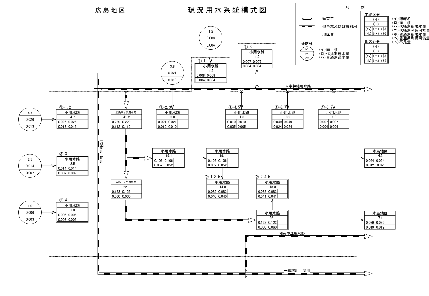
現況用水系統模式図
