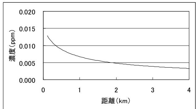
図 5-1-21 接地逆転層崩壊時（フュミゲーション発生時）における短期付加濃度の距離減衰図
