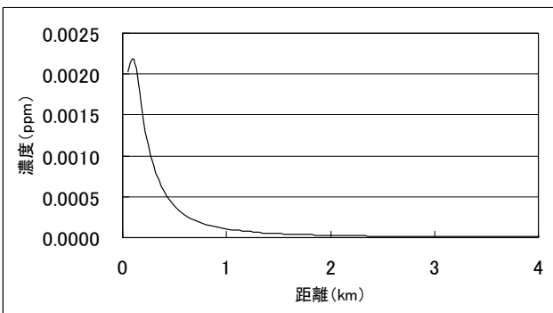
図 5-1-19 大気が不安定な気象条件下における短期付加濃度の距離減衰図
