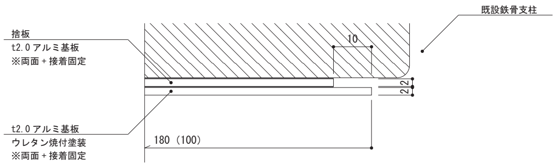
断面図 S=1/1
