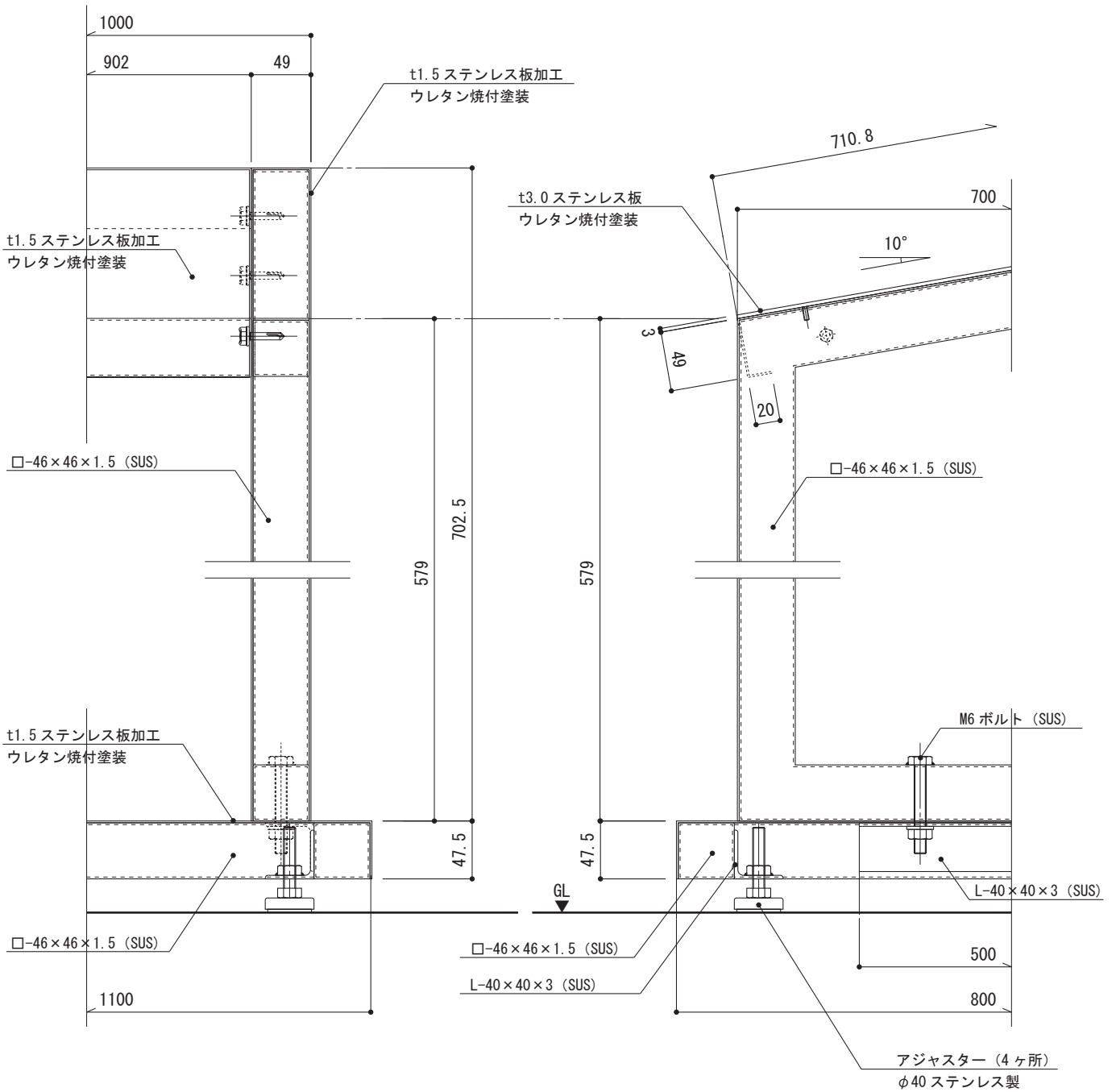
断面図 S=1/5
