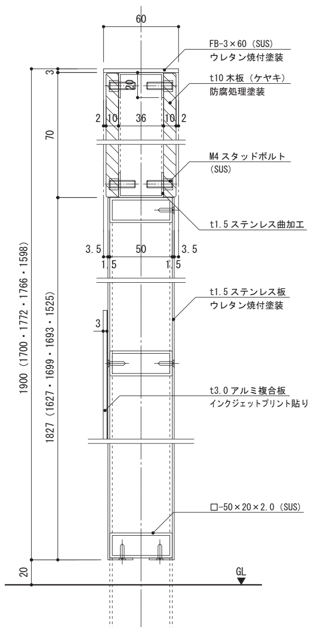
C 断面図 S=1/3
