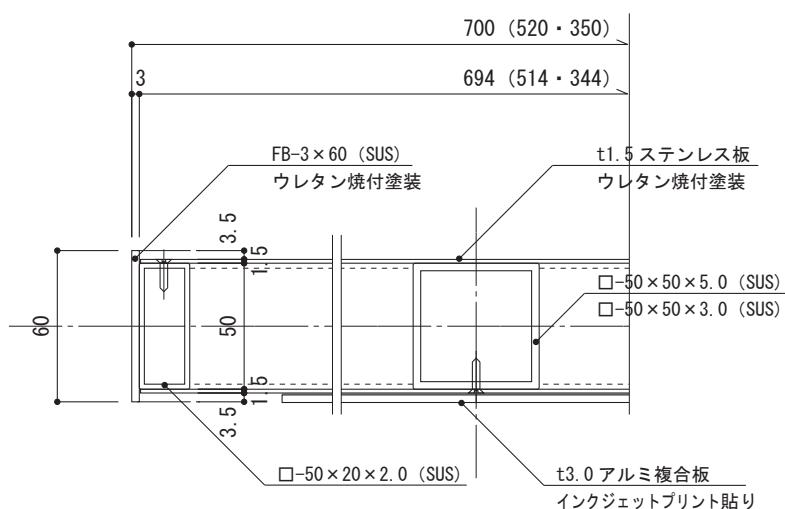
B 断面図 S=1/3
