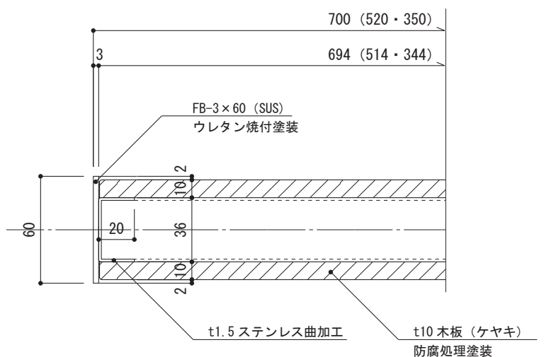
A 断面図 S=1/3
