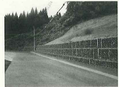
災害防止対策工事の施工例 (清里区青柳地内)
