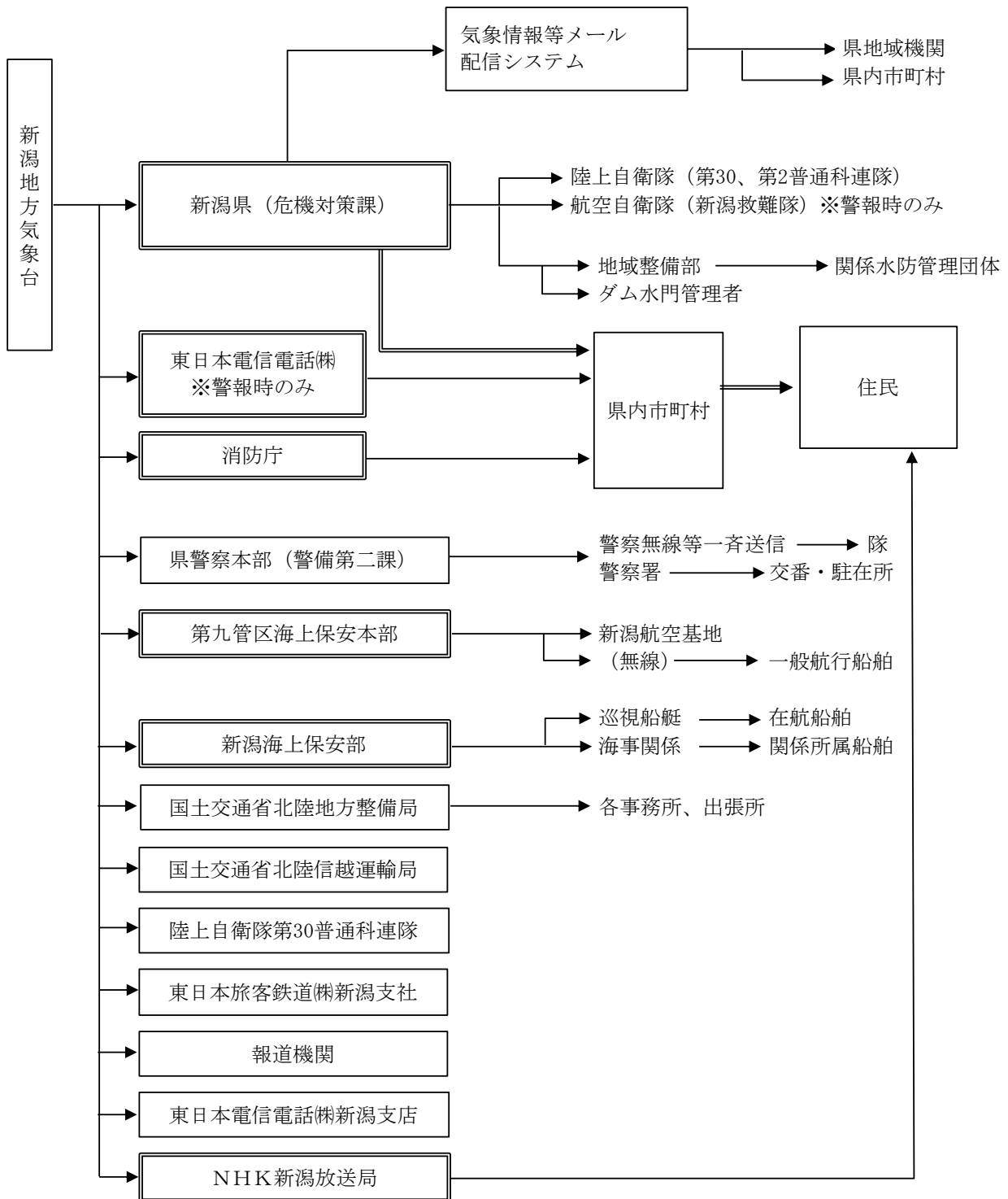
気象警報等の伝達系統図
