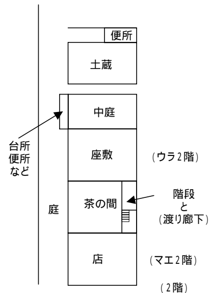
【図1-2-7 町家の間取りの一例】
