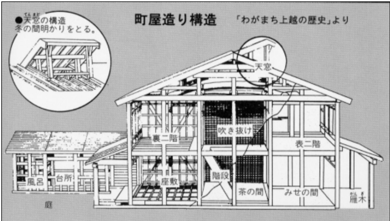
【図 1-3-40 町家造りの構造】
