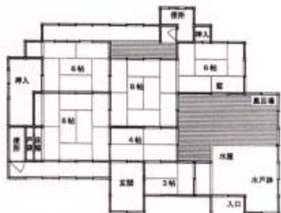
【図1-3-24 小倉佐市郎（250石）邸平面図】
