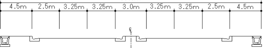
標準横断面図
