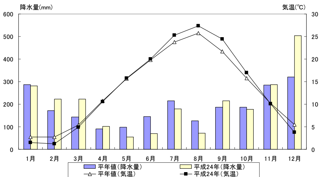
図 2-1-2(1) 平年値及び平成24年の平均気温・降水量（大湊地域気象観測所）
