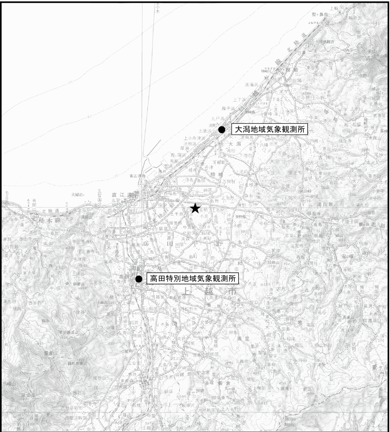
図 2-1-1 気象観測所の位置
