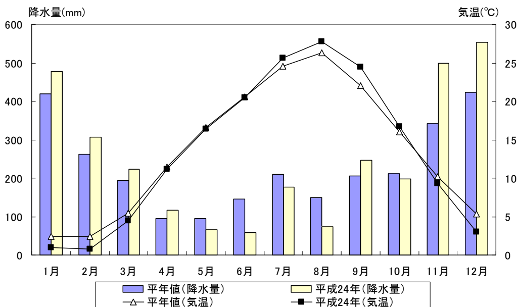
図 2-1-2(2) 平年値及び平成24年の平均気温・降水量（高田特別地域気象観測所）
