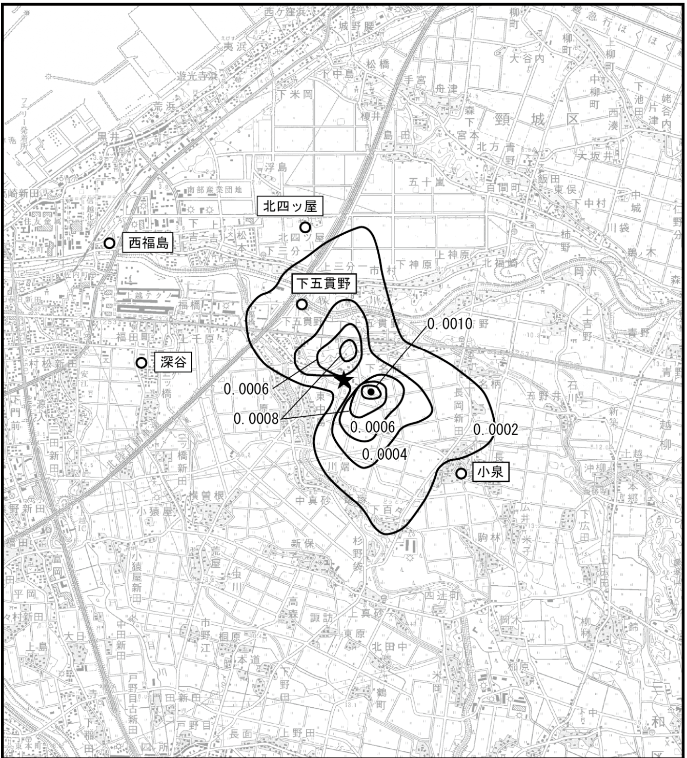
図 5-1-17(1) 施設の稼働に伴うダイオキシン類加濃度 予測結果 (予測ケース: 排ガス量最大)
